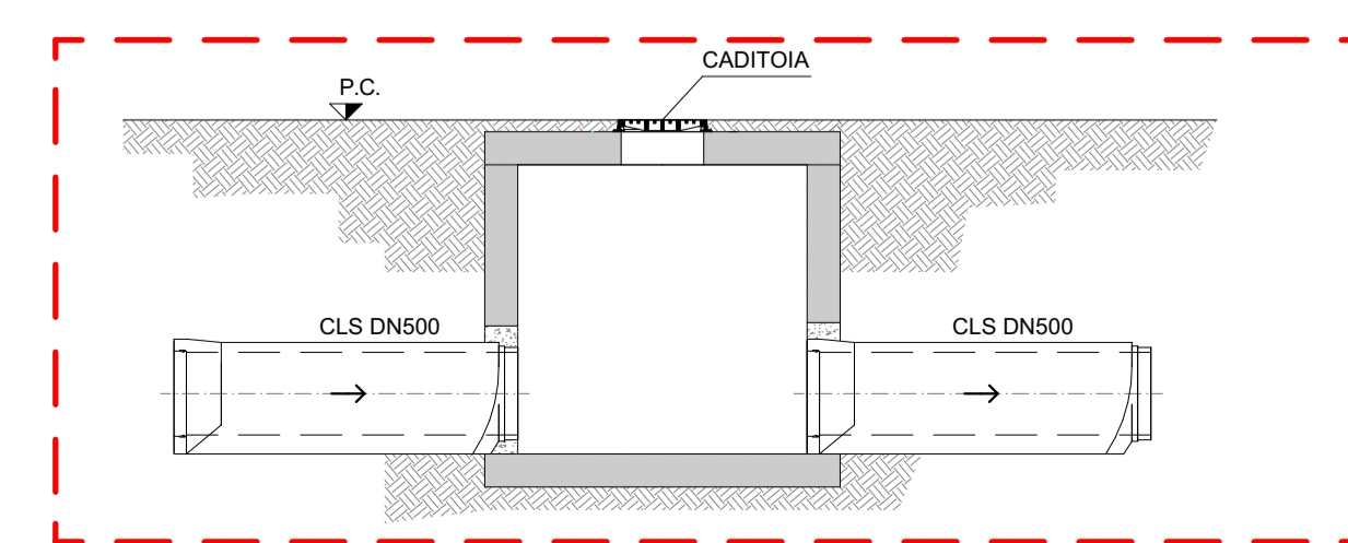
DETTAGLIO 3 - scala 1:50 Pozzetti caditoia tubazioni CLS
