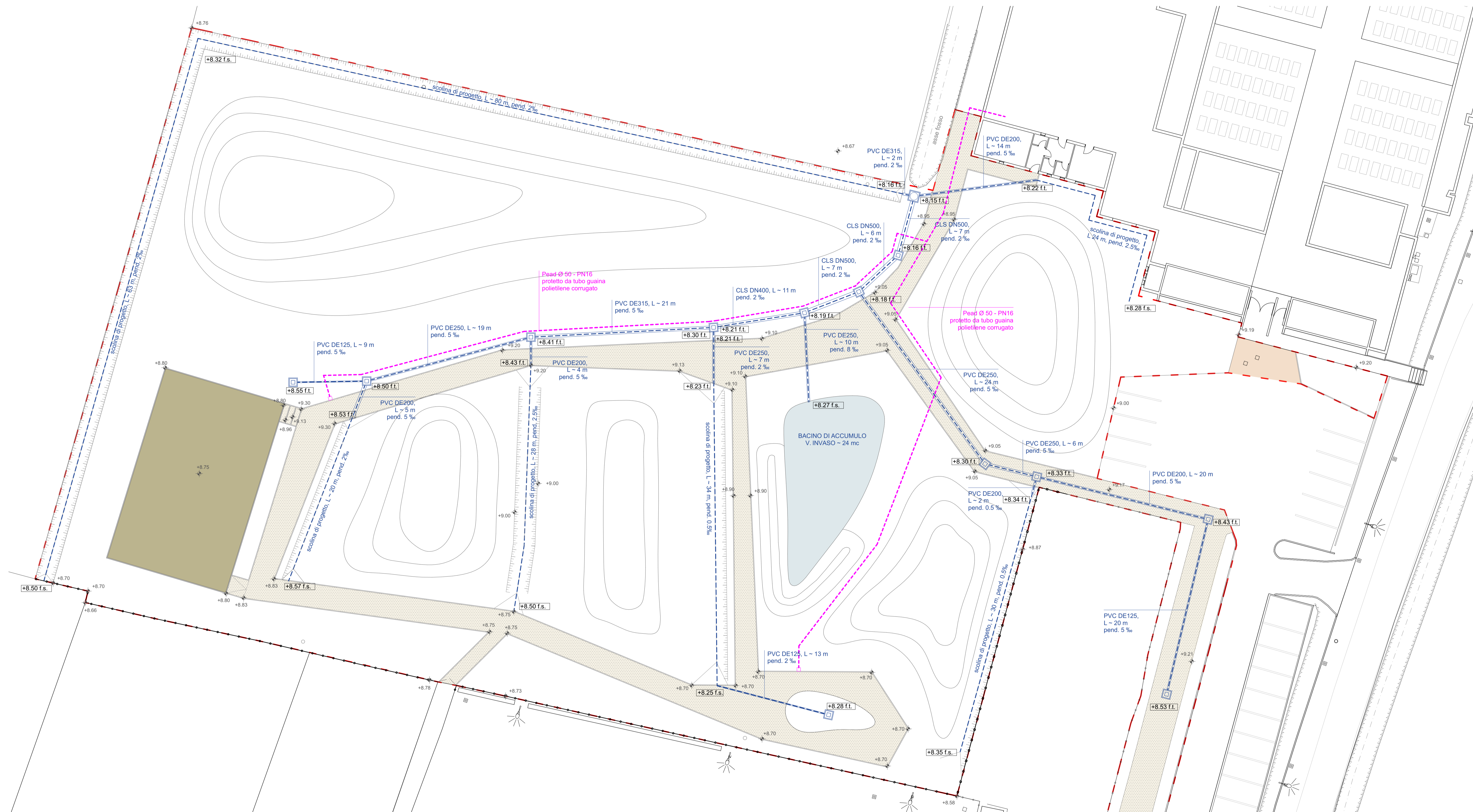
PLANIMETRIA DELLE RETI DI PROGETTO - scala 1:200
