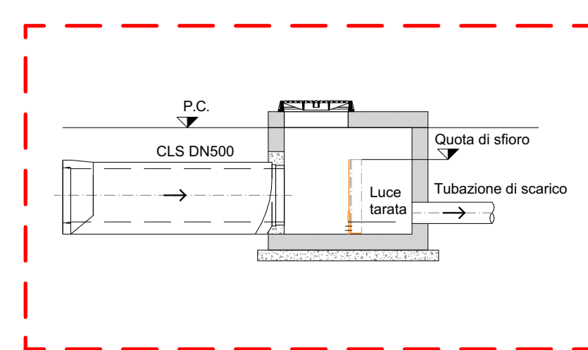
DETTAGLIO 1 - scala 1:50 Pozzetto limitatore di portata
