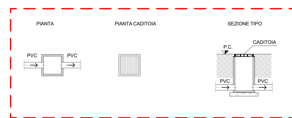
DETTAGLIO 2 - scala 1:50 Pozzetti caditoia tubazioni PVC
